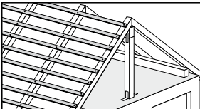
Battens
